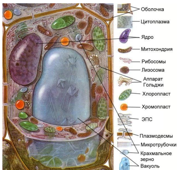
Рис. 3. Элементы клетки
